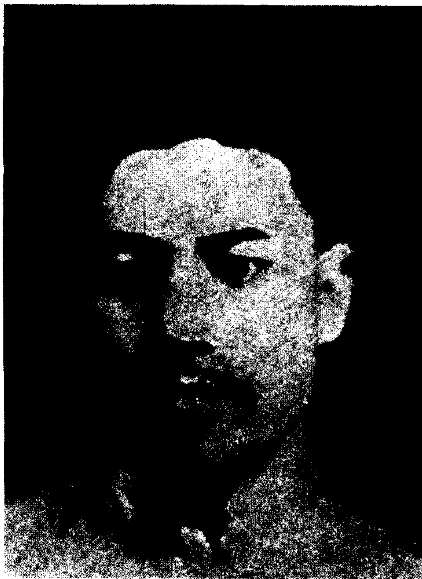
于 方 舟
